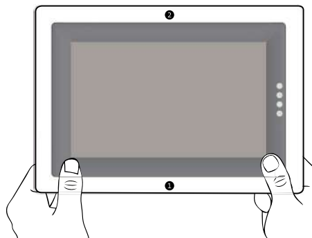
BT 800: Ausklipsen des Frontrahmens
